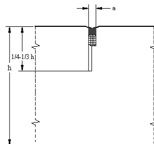
Rys. Szczelina przeciwskurczowa
